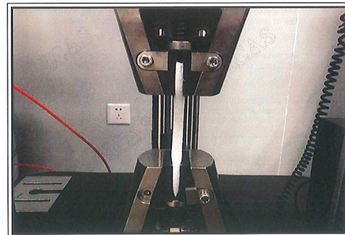
拉伸试验中
