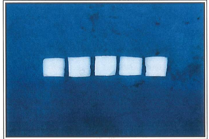
压缩永久变形试验后
