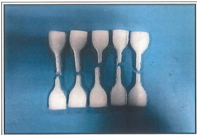
拉伸试验后
